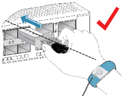
SFP+ 电缆拆卸示意图 Figure: Remove SFP+ Cable
